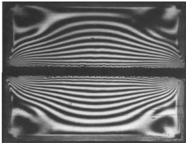
Рис. 1 и 2. Результат экспериментального исследования: распределение контактных напряжений вдоль контактной линии БПА при усадке и при расширении цементов (в данном эксперименте БПА с оплеточной нитью). На рисунке хорошо видно существенная концентрация напряжений на поверхности БП арматуры, по сравнению предыдущим экспериментом (Исследования проводились в закрытой лаборатории завода «БОЛЬШЕВИК» 1988 г.)
