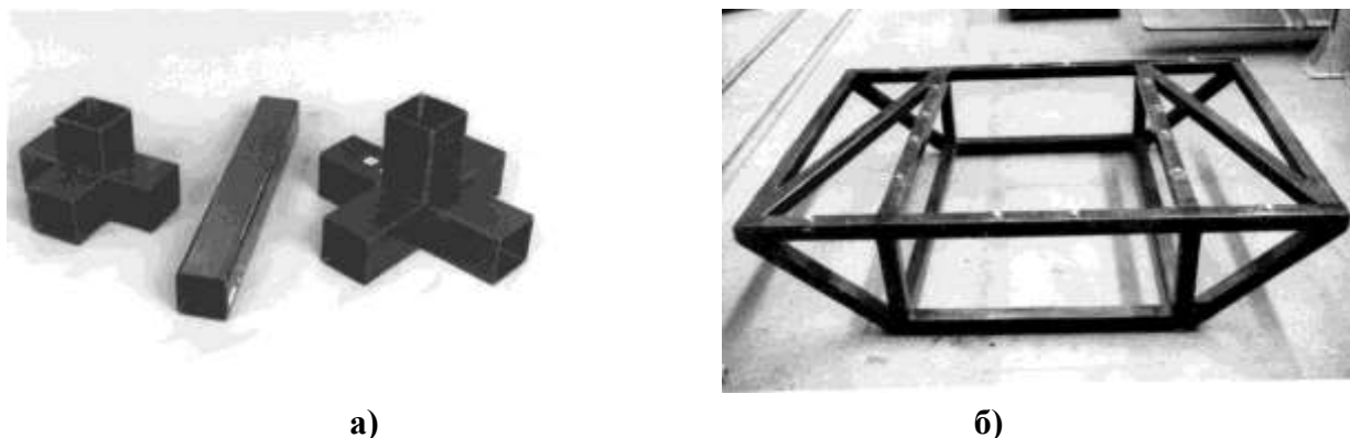
Рис. 2. Трубчатый элемент с фитингами (а) и ферменная конструкция (б), изготовленные методом автоматизированной намотки
