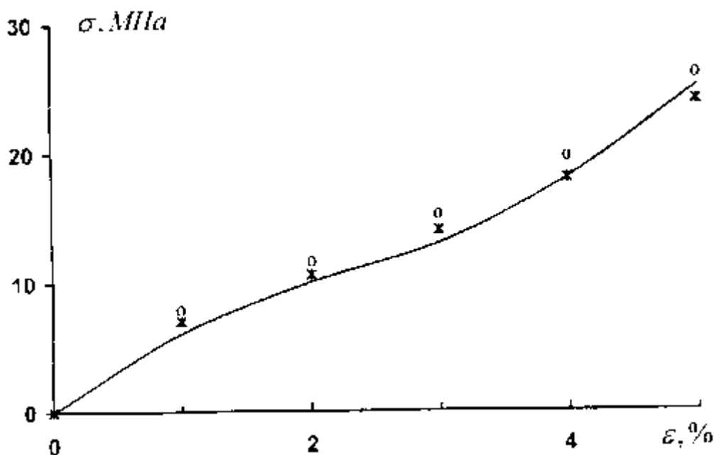
Рисунок 1 - Диаграмма растяжения лавсановой нити, T = 20^\circ C при скорости деформирования \dot{\varepsilon} = 0,083 c^{-1} (сплошная линия - эксперимент, о - расчет до коррекции,
